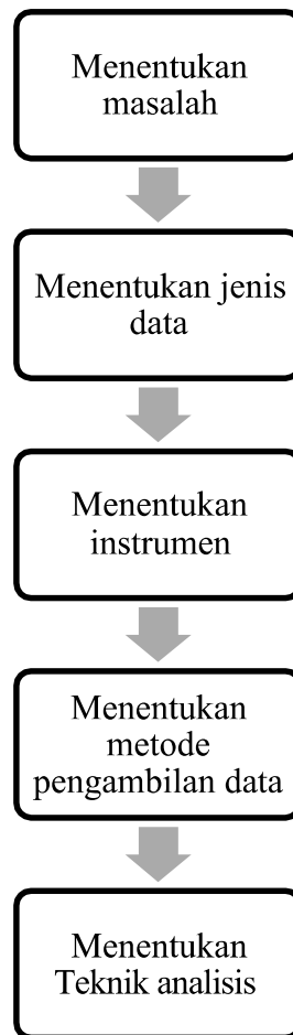
Gambar 3.2 Desain Penelitian
