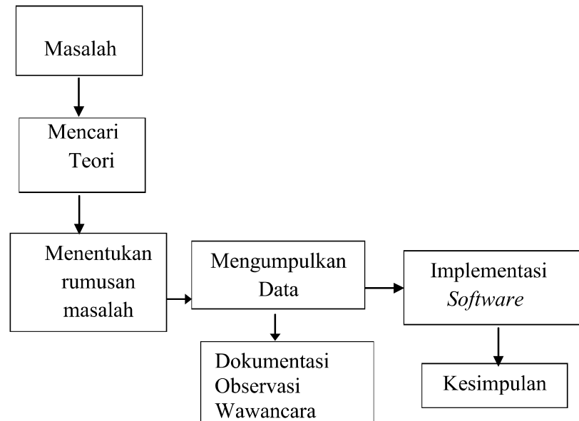
Gambar 3.1 Desain Penelitian
