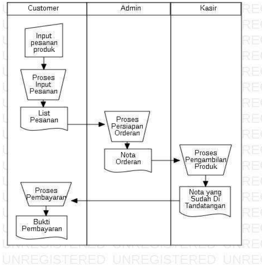
Gambar 3. 5. Aliran sistem yang sedang berjalan
