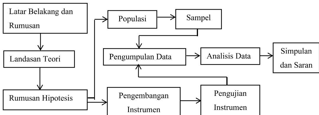
Gambar 3.1 Desain Penelitian
