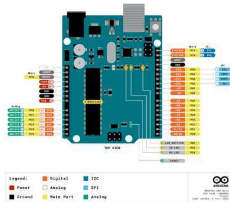
Gambar 2. 9 Pin Out Arduino Uno
