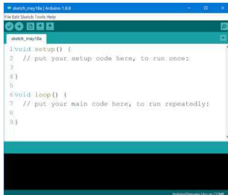
Gambar 2. 17 Arduino Ide
