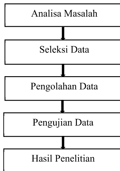
Gambar 3. 1 Desain Penelitian
