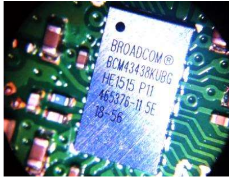
Gambar 2.7 Radio Nirkabel (Sumber : Peneliti)
