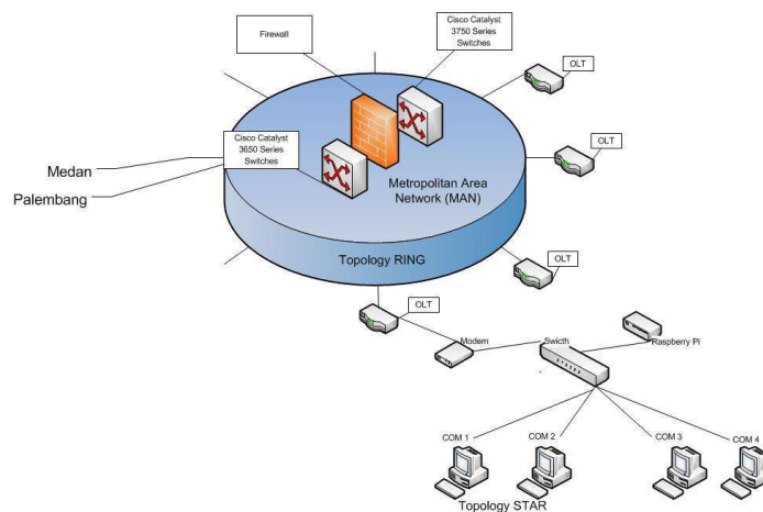
Gambar 3.6 Topologi yang di usulkan (Sumber : Peneliti)
