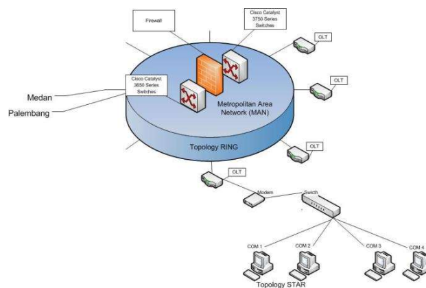
Gambar 3.2 Topologi Yang Sedang Berjalan (Sumber : Peneliti)
