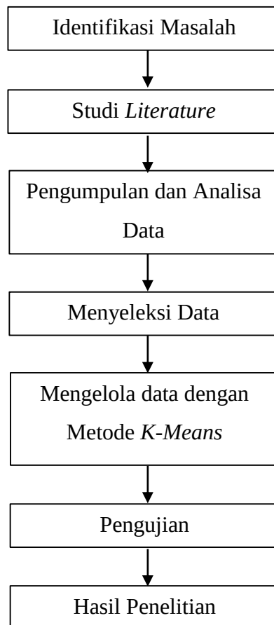
Gambar 3.1. Desain Penelitian
