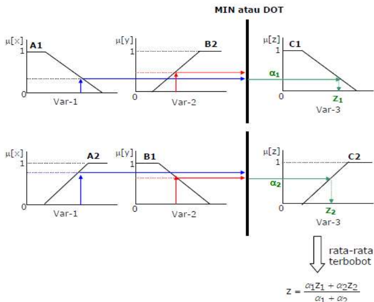
Gambar 2.14 Inferensi dengan Menggunakan Metode Tsukamoto
