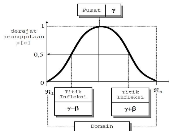
Gambar 2.10 Karakteristik Fungsional Kurva PI
