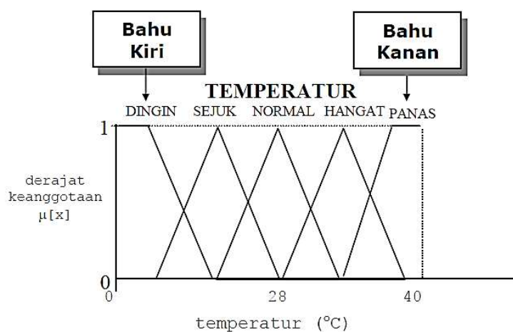
Gambar 2.7 Kurva Bentuk Bahu
