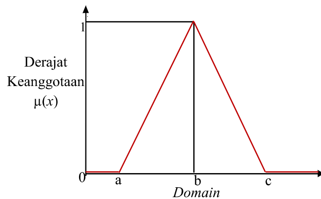
Gambar 2.5 Representasi Kurva Segitiga
