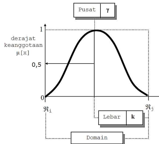
Gambar 2.12 Karakteristik Fungsional Kurva GAUSS
