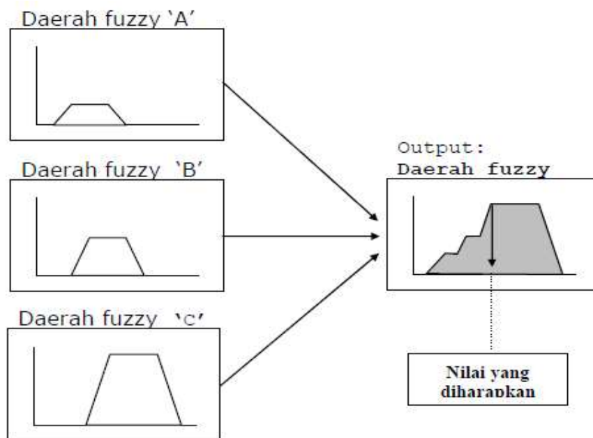
Gambar 2.13 Proses Defuzzyfikasi
